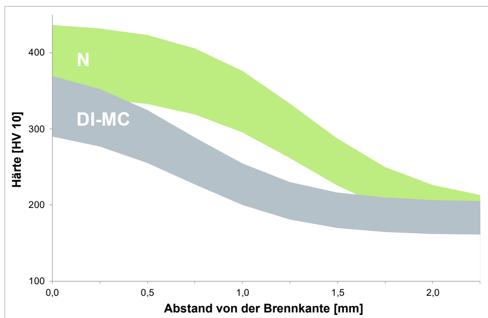
Aufhärtung von DI-MC 355/S355ML an der Schnittkante beim Sauerstoff-Acetylen-Brennschneiden im Vergleich mit normiertem S355N
