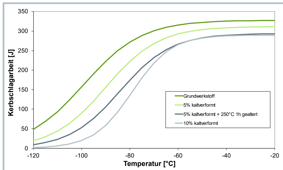
Beispielhafter Einfluss von Kaltverformung und Alterung auf die Kerbschlagarbeit-Temperatur-Kurve von DI-MC 355 T/S355ML (Mittelwertkurven ohne Darstellung von Streuung)
