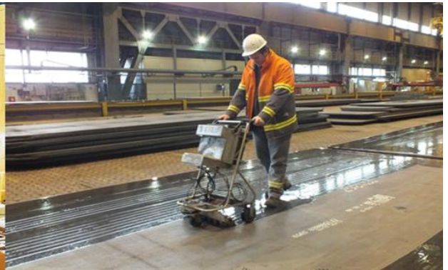
Manuelle Ultraschallprüfung für Blechdicken bis zu 400 mm
