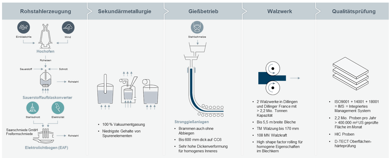
Schema : Produktionsprozess von DILLINGER
