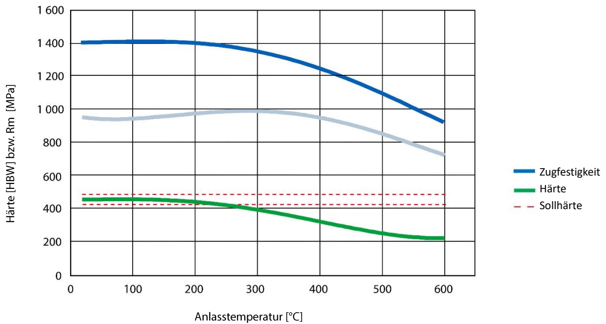
Grafik 5 Typische Eigenschaften von DILLIDUR 450 nach dem Anlassen und Abkühlen auf Raumtemperatur (Anhaltswerte für 20 mm)
