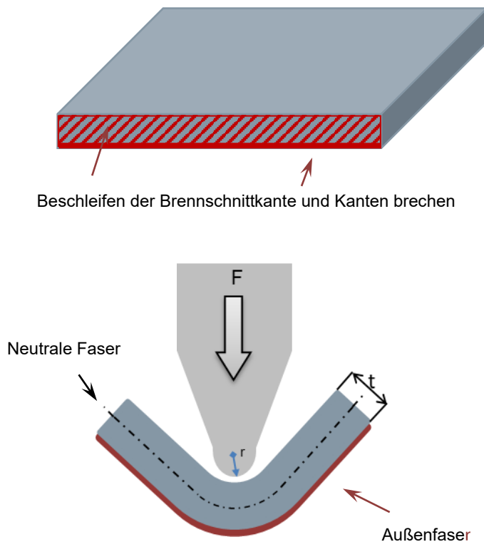
Grafik 2 Bearbeiten einer Schnittkante und Dehnung an der Außenfaser
