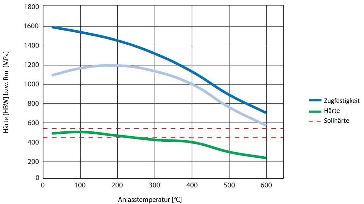
Grafik 6 Typische Eigenschaften von DILLIDUR 500 nach dem Anlassen und Abkühlen auf Raumtemperatur (Anhaltswerte für 20 mm)
