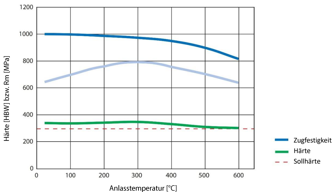
Grafik 3 Typische Eigenschaften von DILLIDUR 325 L nach dem Anlassen und Abkühlen auf Raumtemperatur (Anhaltswerte für 10 mm bei einer Haltezeit von 30 Minuten)
