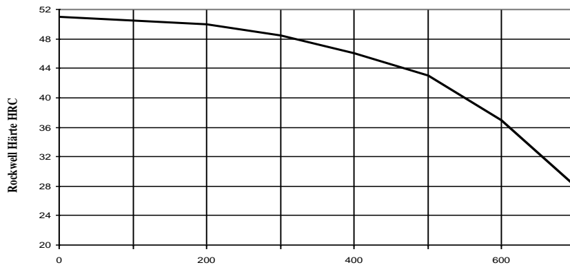
Anlasstemperatur [°C] (Haltedauer 1 h, Luftkühlung) Hinweis: Diagrammwerte sind Mittelwerte an Proben Durchmesser 25 mm, Länge 50 mm, gehärtet bei 850 °C in Öl
