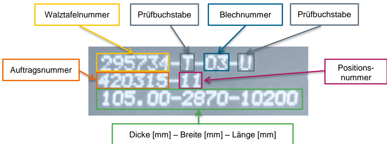
Abbildung 3: DF Standard-Farbbeschriftung (schematisch)
