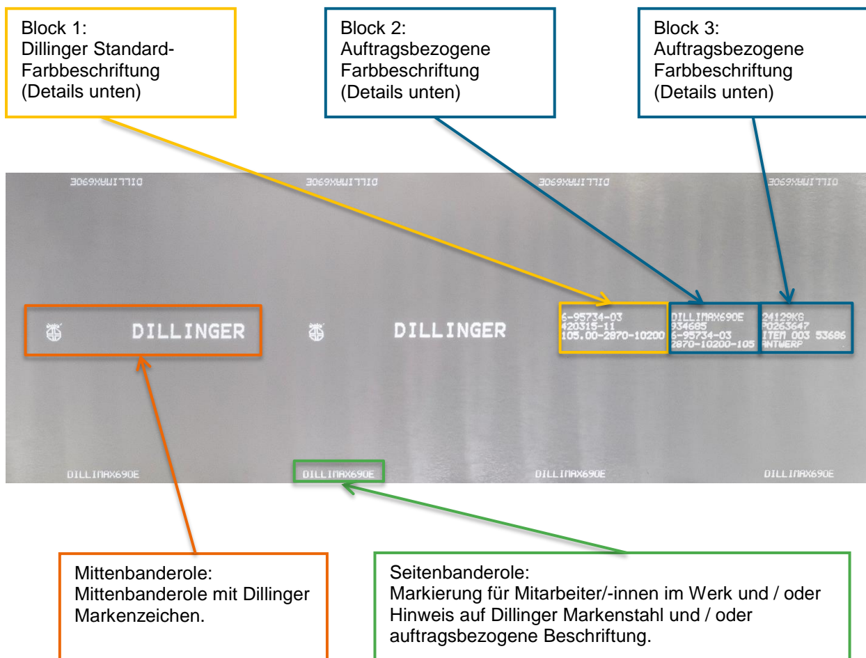
Abbildung 1: Aufbau der Dillinger Farbbeschriftung (schematisch)
